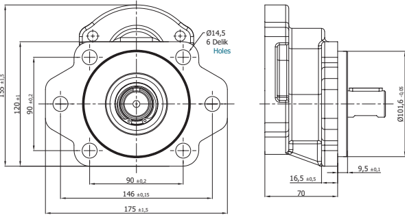
SAE 'B' 2-4 BOLTS D2
