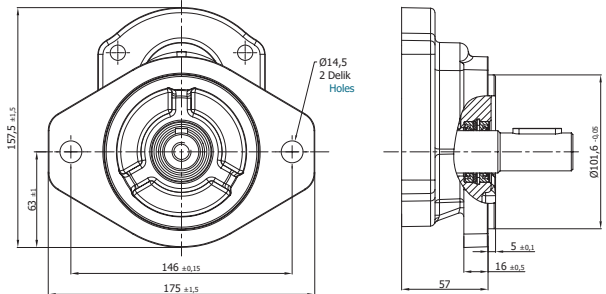
SAE 'B' 2 BOLTS K
