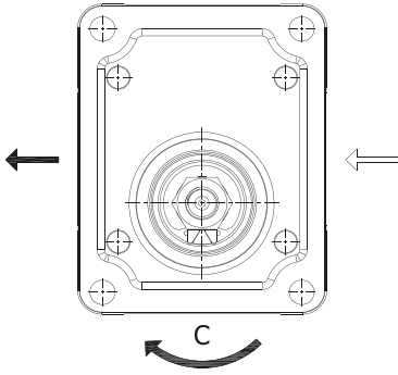
Sağ Döndürlü Pompa Clockwise Rotation
