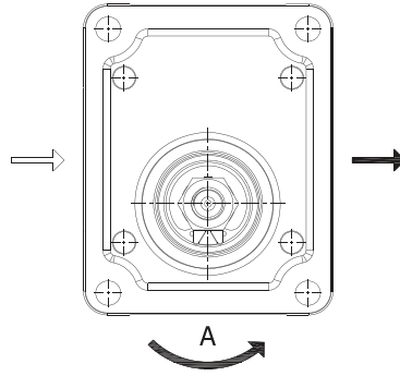
Sol Döndürlü Pompa Counter-clockwise Rotation
